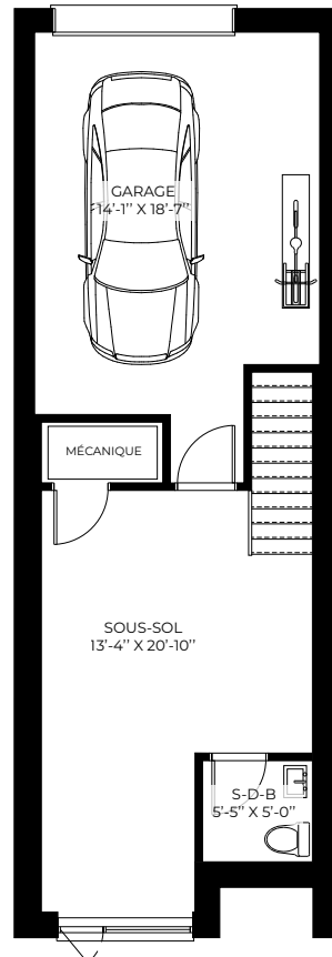
Sous-sol (679 pi 2 )
